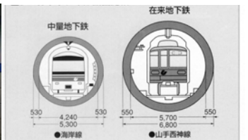
トンネルの大きさの比較
